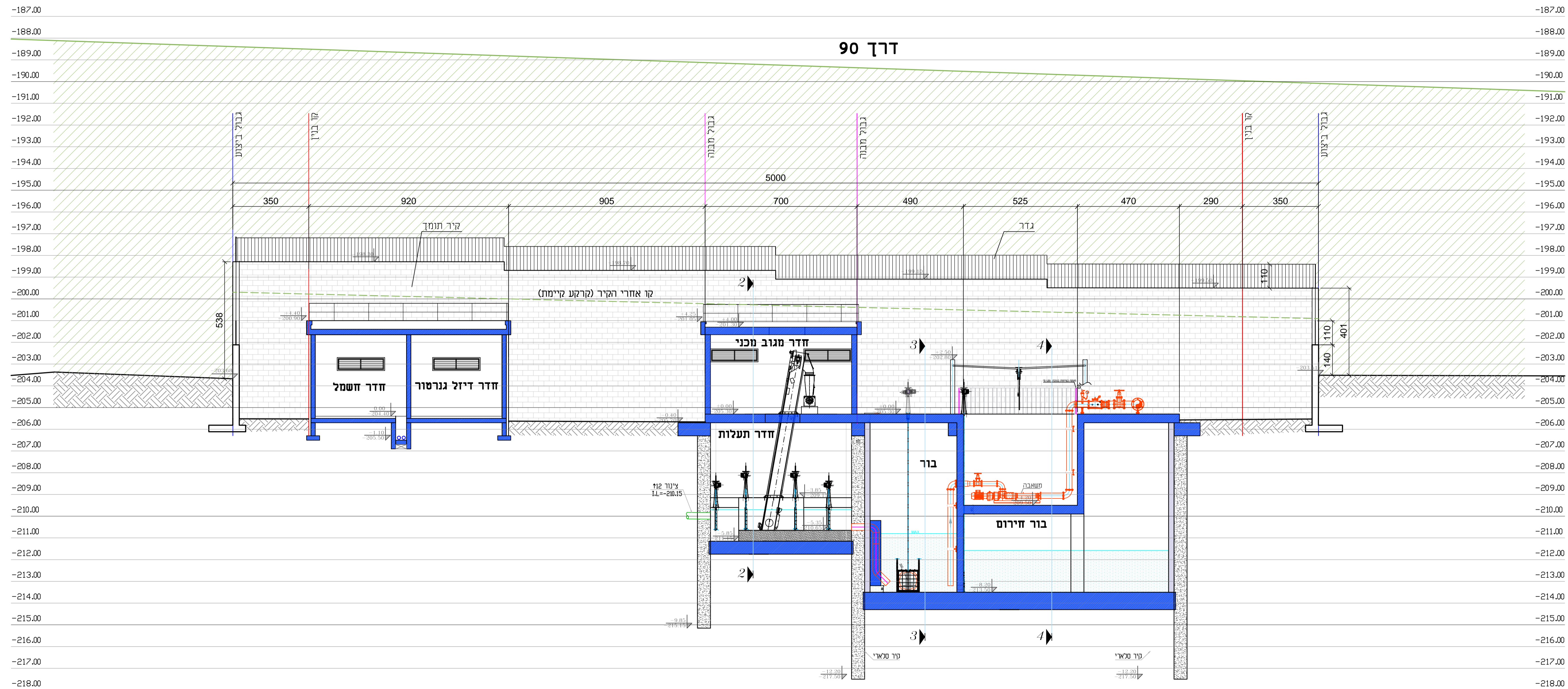
חתך ג-ג קנ"מ 1:100
