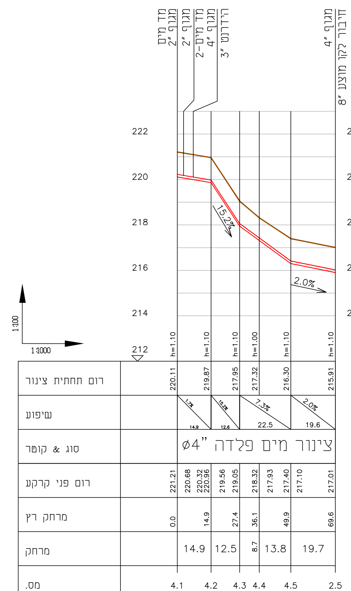
1:100/1:1000 - קו צינור: 4
