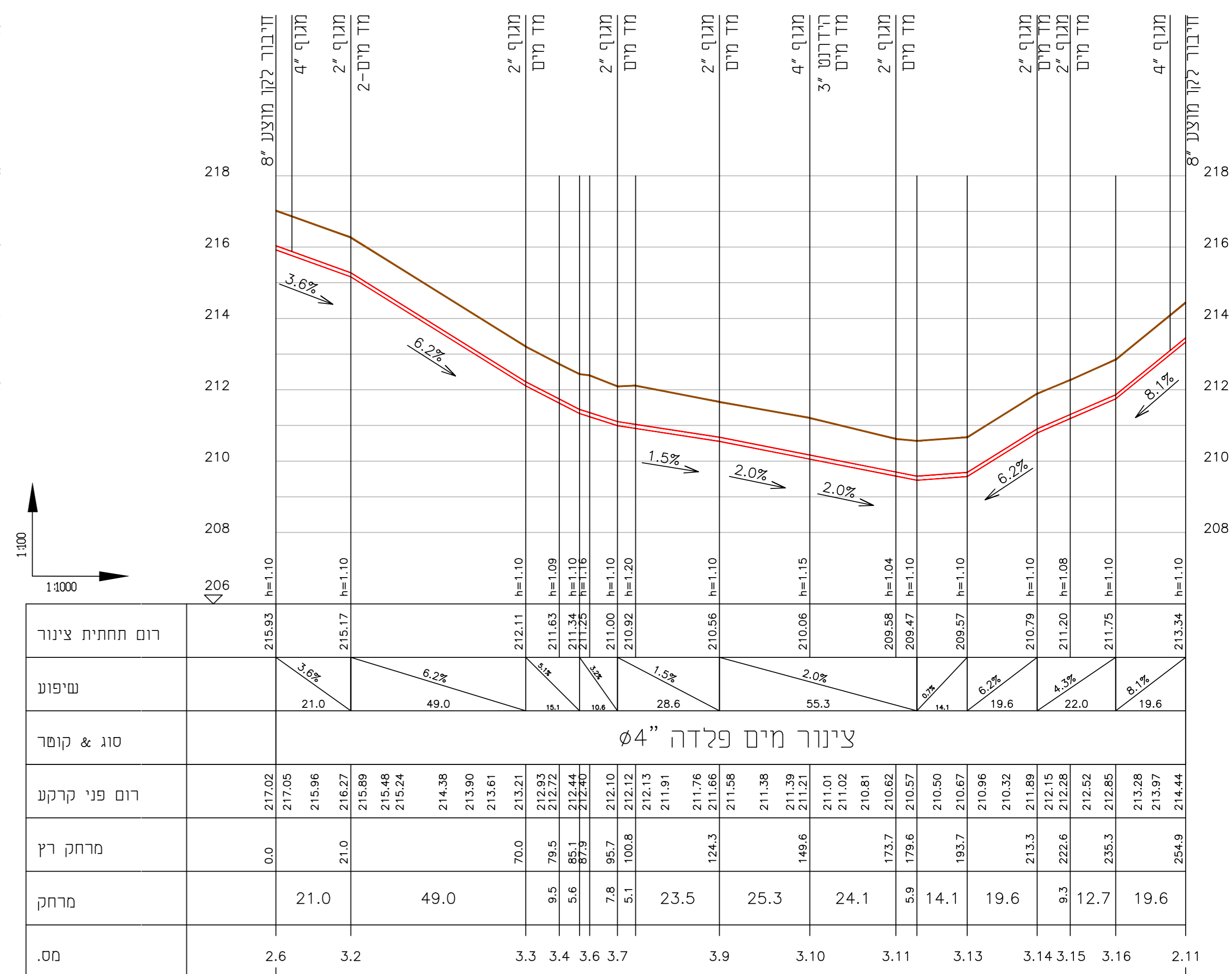
1:100/1:1000 - קו צינור: 3
