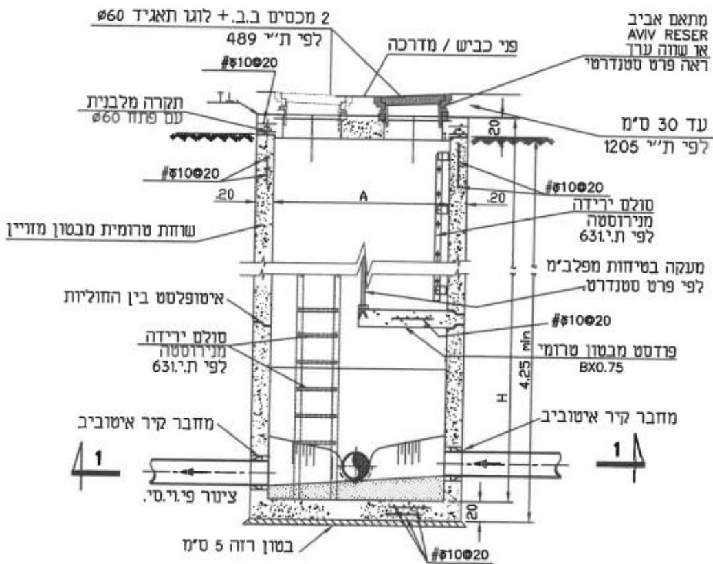
חתך 2-2
