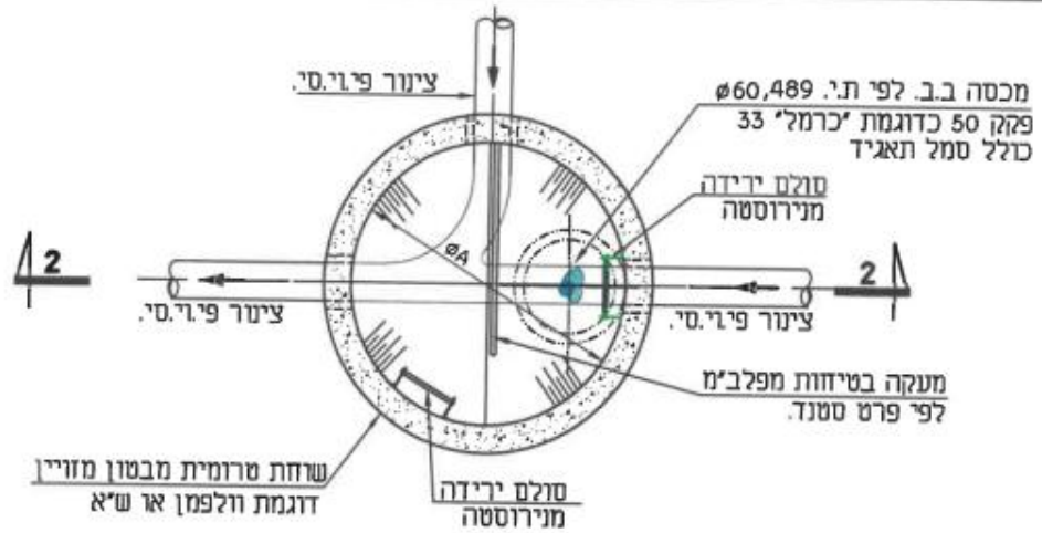
חתך 1-1
