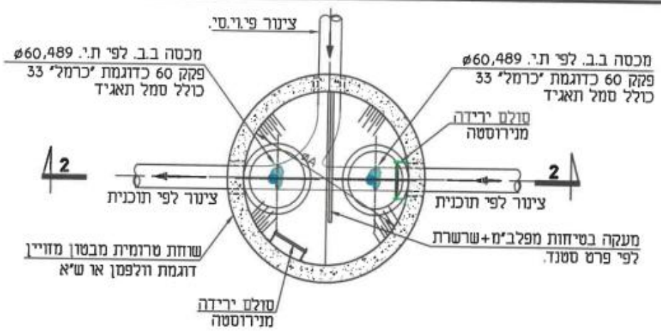
חותך 1-1
