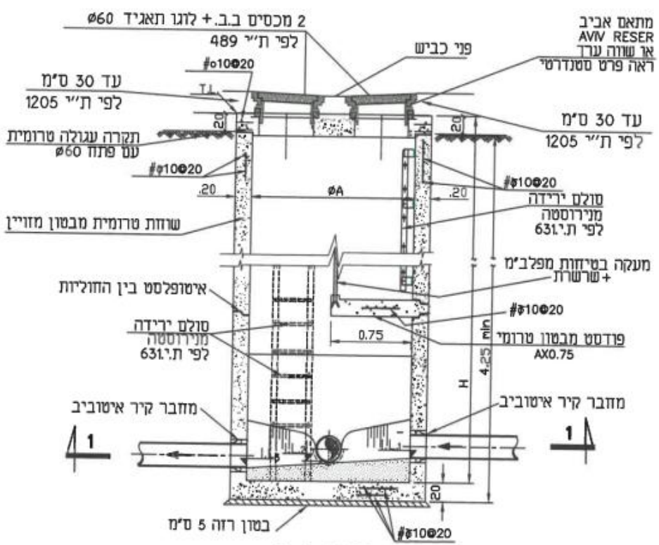
חותך 2-2
