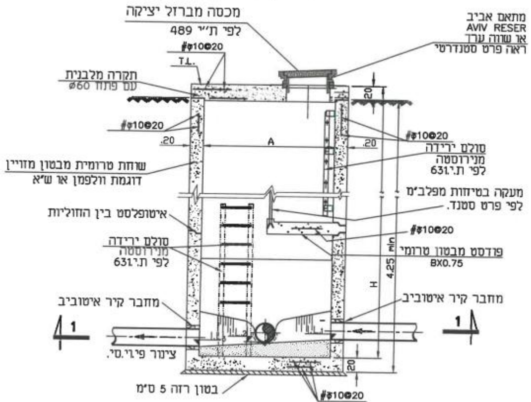
חתך 2-2
