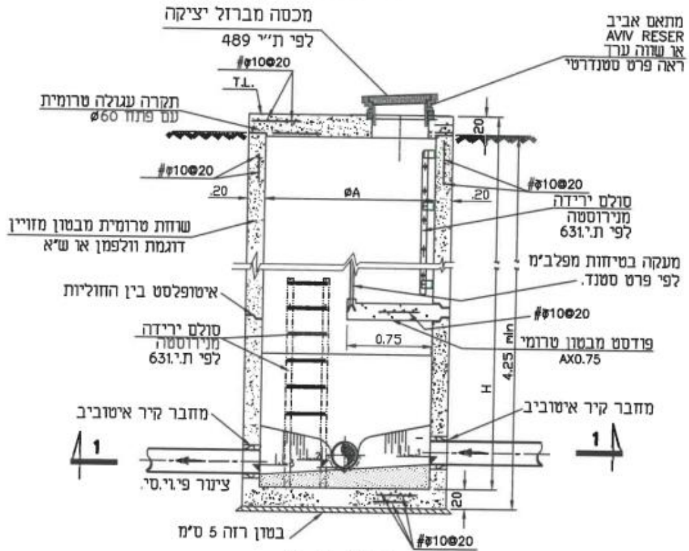
חתך 2-2
