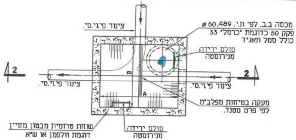
חתך 1-1
