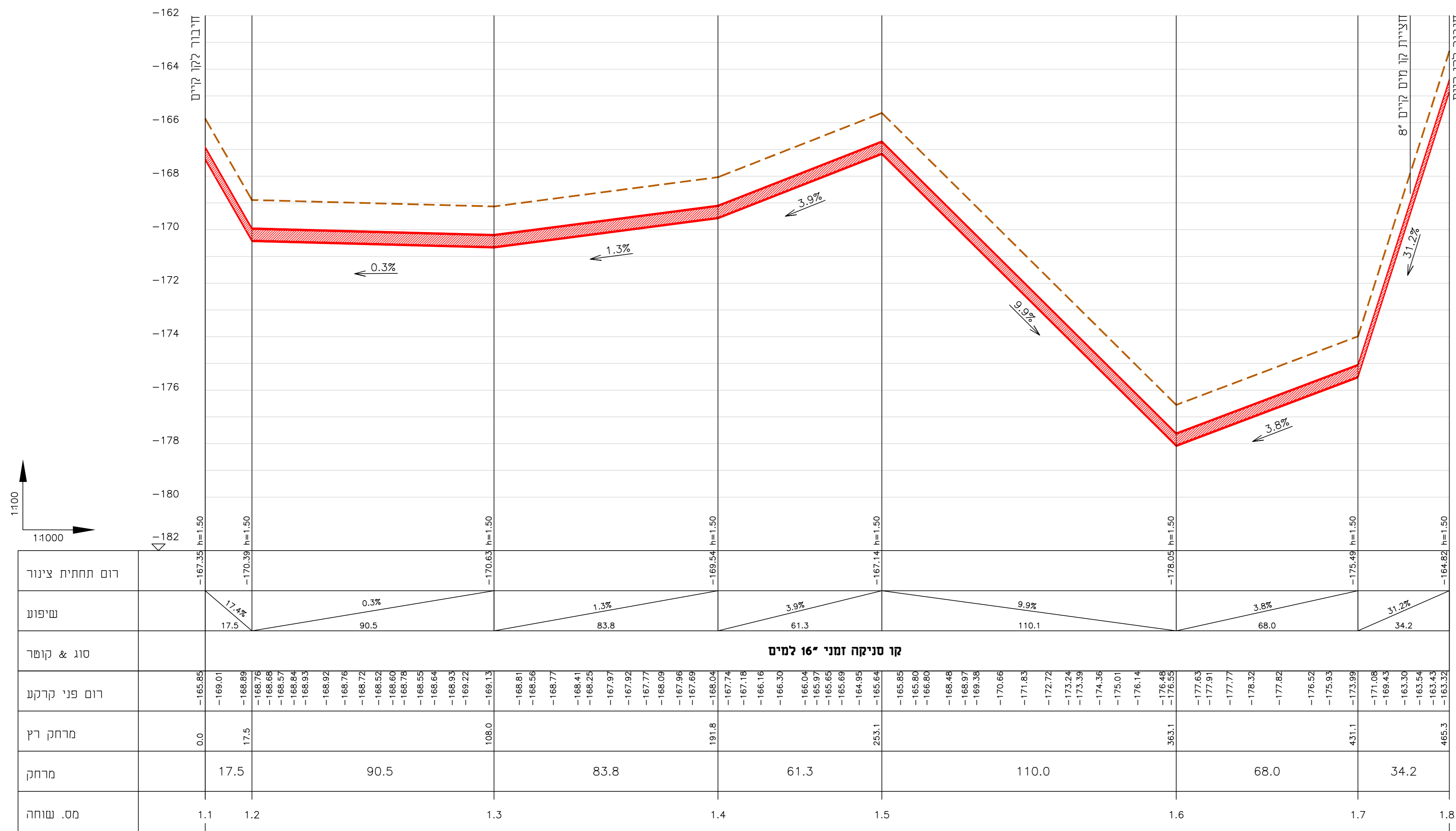
1 קו צינור: 1 - 1:100/1:1000
